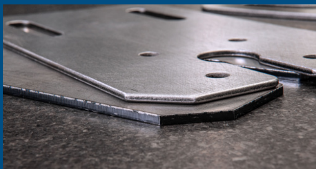
Peças de corte laser antes e depois de processadas na EdgeBreaker® 6000.
